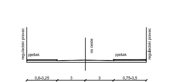
KARAKTERISTIČAN POPREČNI PRESJEK C - C M 1:200
