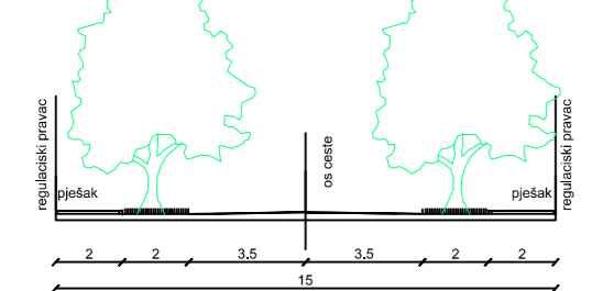
KARAKTERISTIČAN POPREČNI PRESJEK A - A M 1:200
