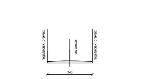
KARAKTERISTIČAN POPREČNI PRESJEK H - H M 1:200
