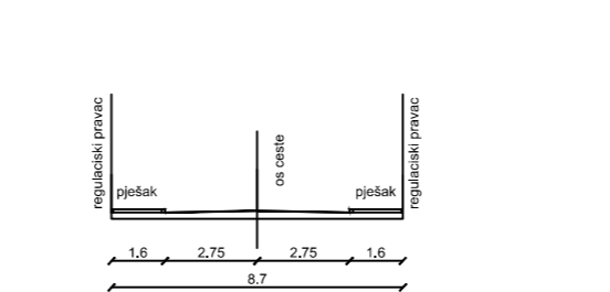
KARAKTERISTIČAN POPREČNI PRESJEK E - E M 1:200
