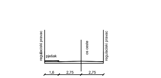
KARAKTERISTIČAN POPREČNI PRESJEK F - F M 1:200
