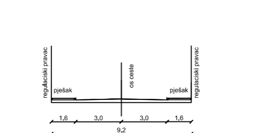
KARAKTERISTIČAN POPREČNI PRESJEK D - D M 1:200
