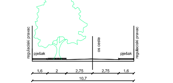
KARAKTERISTIČAN POPREČNI PRESJEK B - B M 1:200
