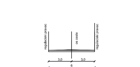
KARAKTERISTIČAN POPREČNI PRESJEK G - G M 1:200
