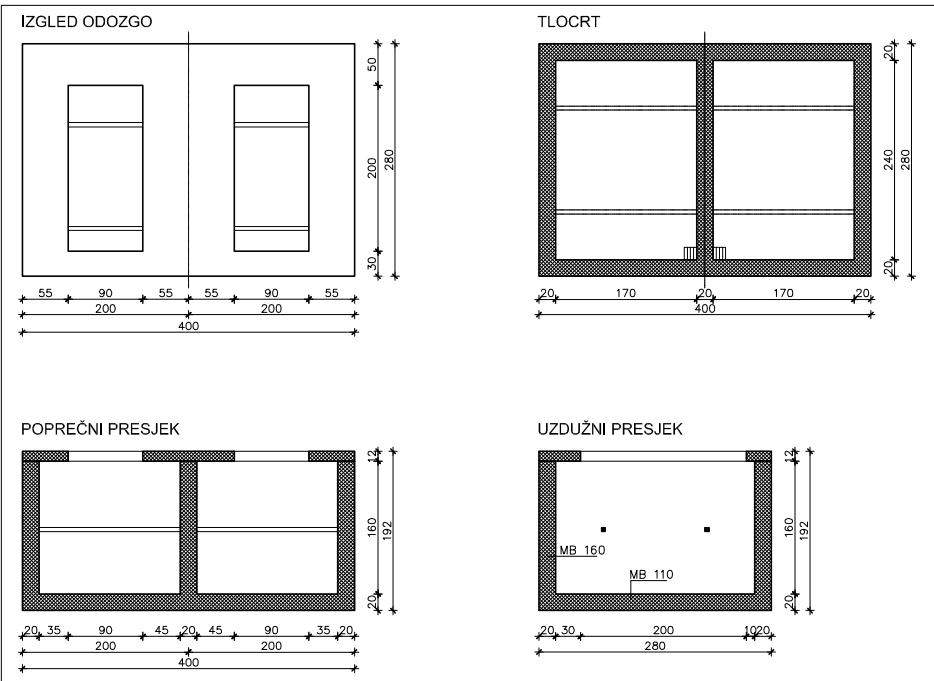
grobnica za 2 x 4 lijesa mj. 1:50
