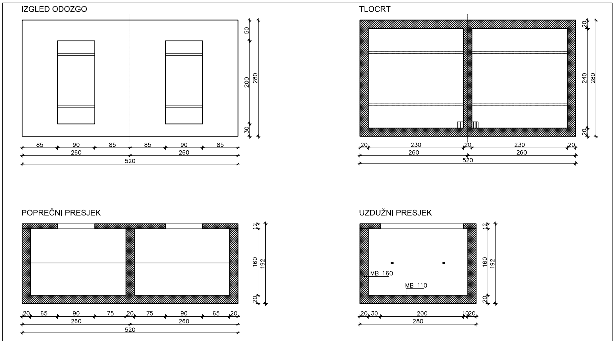
grobnica za 2 x 6 lijesova mj. 1:50
