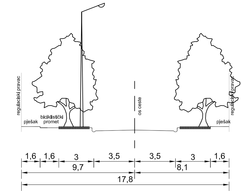
MJ 1: 200 KARAKTERISTIČAN POPREČNI PRESJEK A - A
