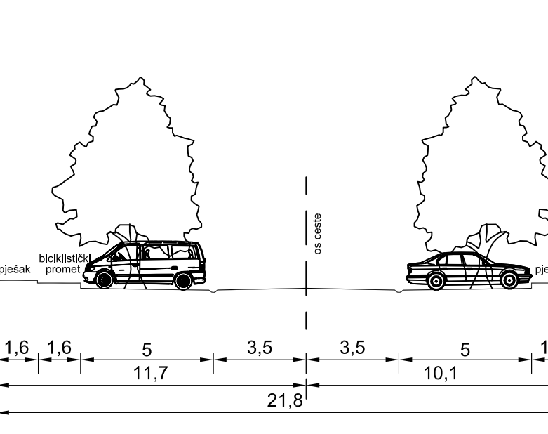
KARAKTERISTIČAN POPREČNI PRESJEK B - B
