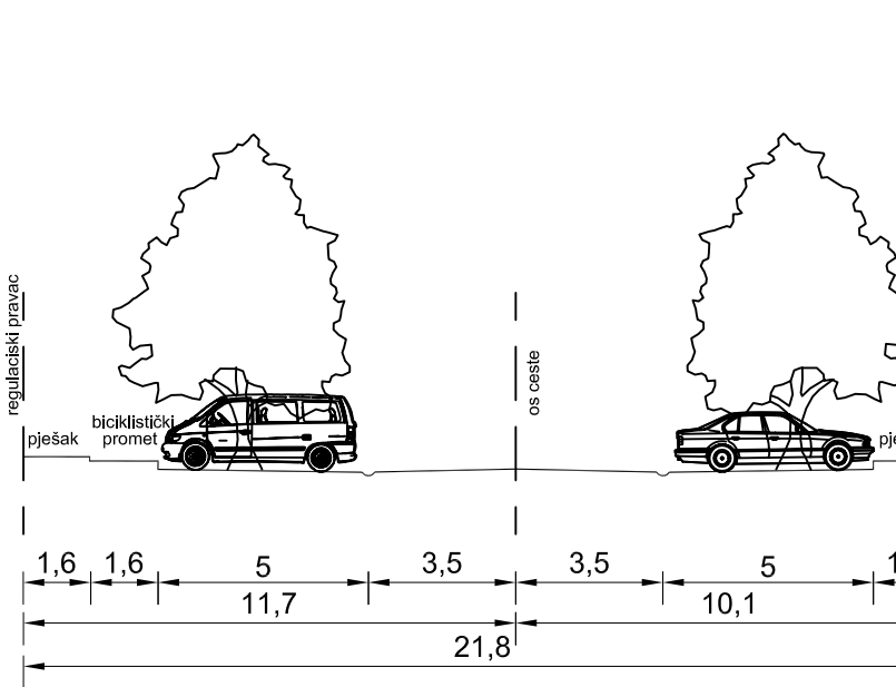
KARAKTERISTIČAN POPREČNI PRESJEK B - B
