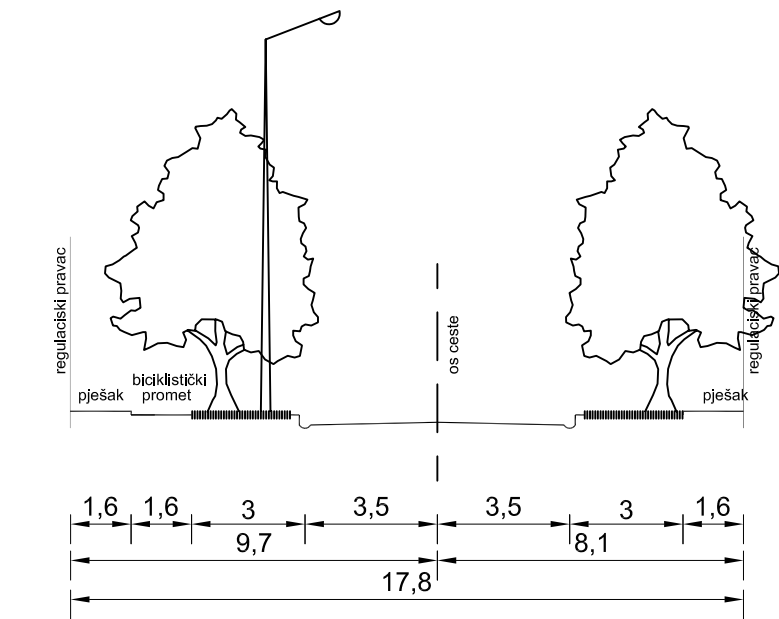
KARAKTERISTIČAN POPREČNI PRESJEK A - A
